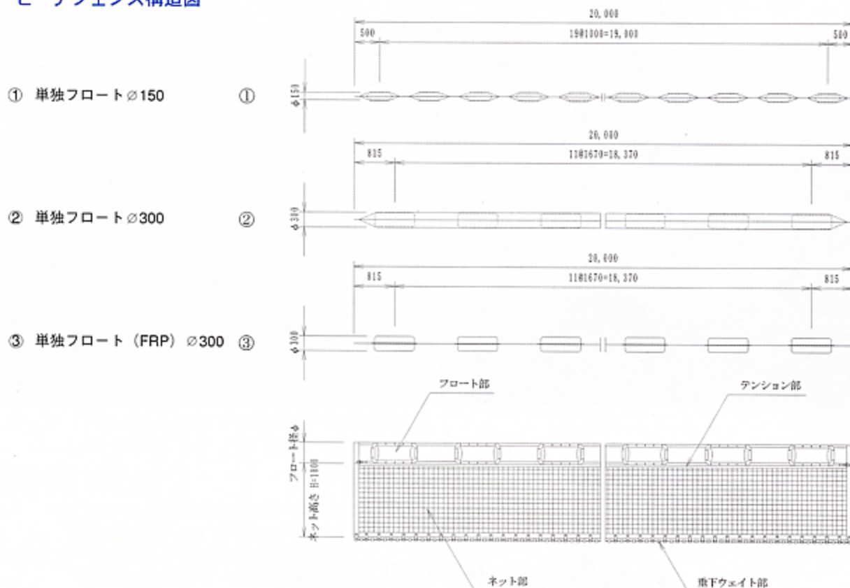
ビーチフェンス構造図
