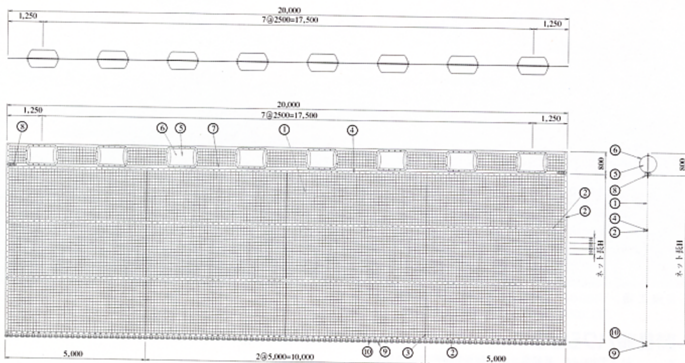
シャークフェンス構造図
